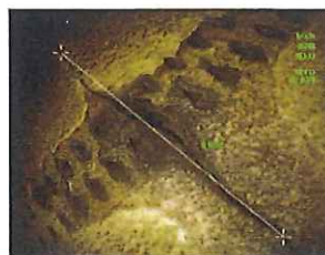
サンプル画像: タービンの割れ
