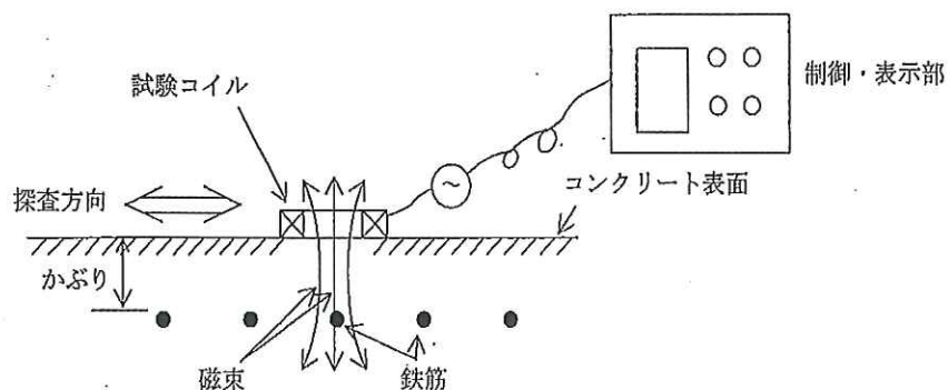
電磁誘導法による鉄筋探査例
