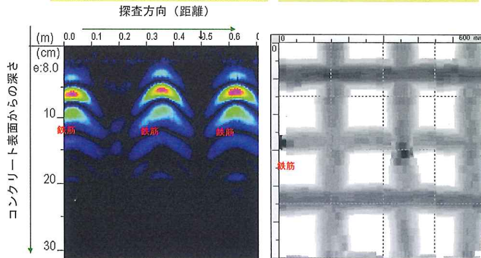
電磁波レーダ法による鉄筋探査例
