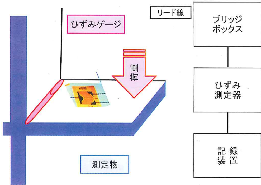
ひずみ測定システムの例
