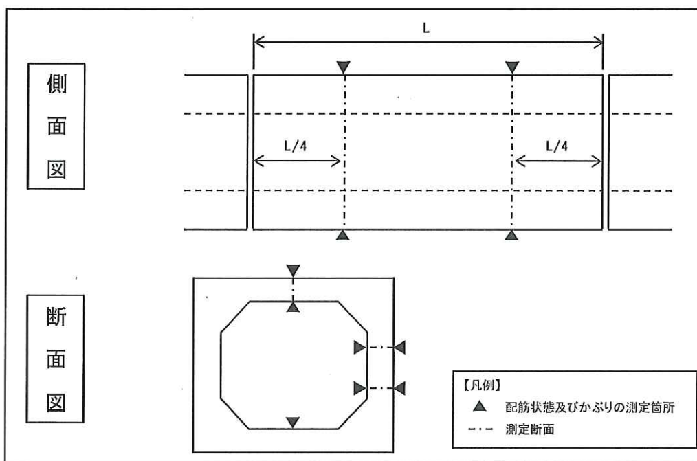
図 7 ボックスカルバートの測定位置（例）
